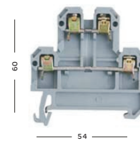
双层端子 厚度6
