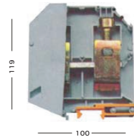
普通型接线端子 厚度31
