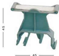
分类标记座 厚度9.5
