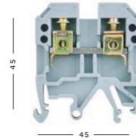
普通型接线端子 厚度8
